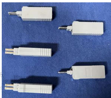
保安、测试接线排
